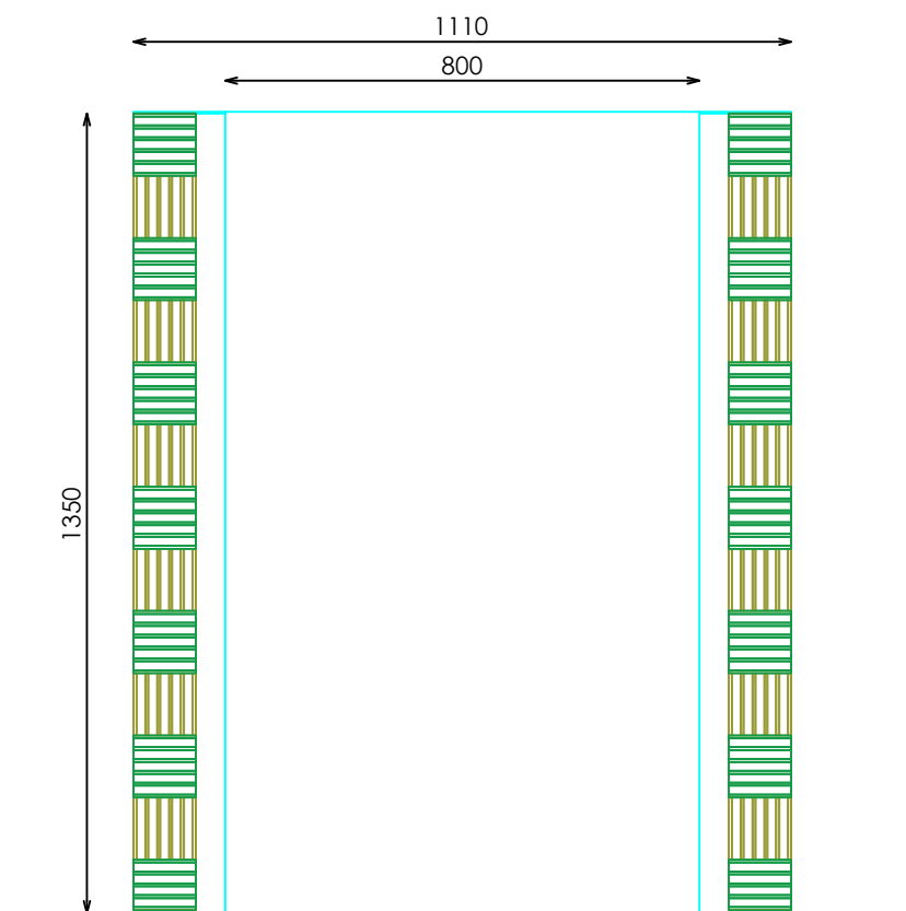
ALZADO TRASERO
