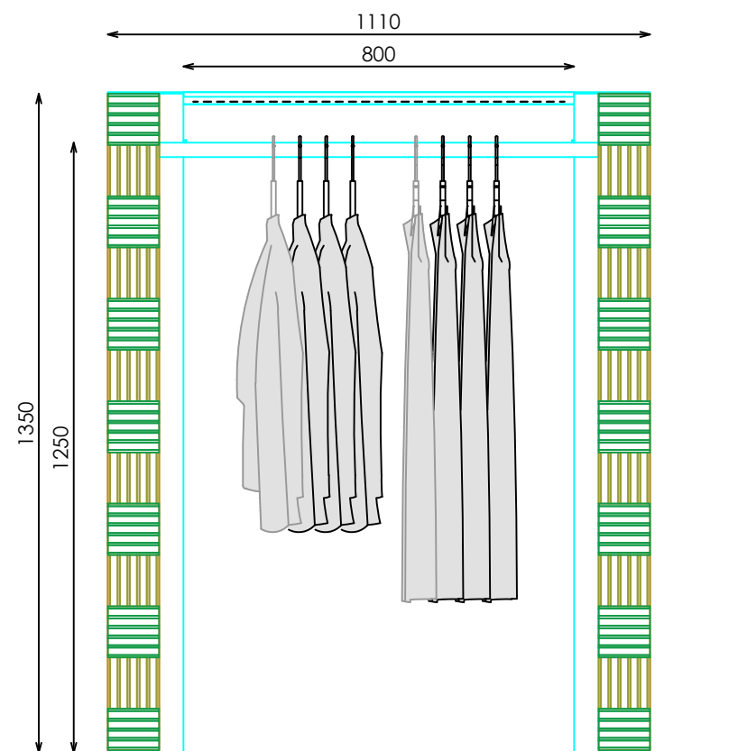
ALZADO
