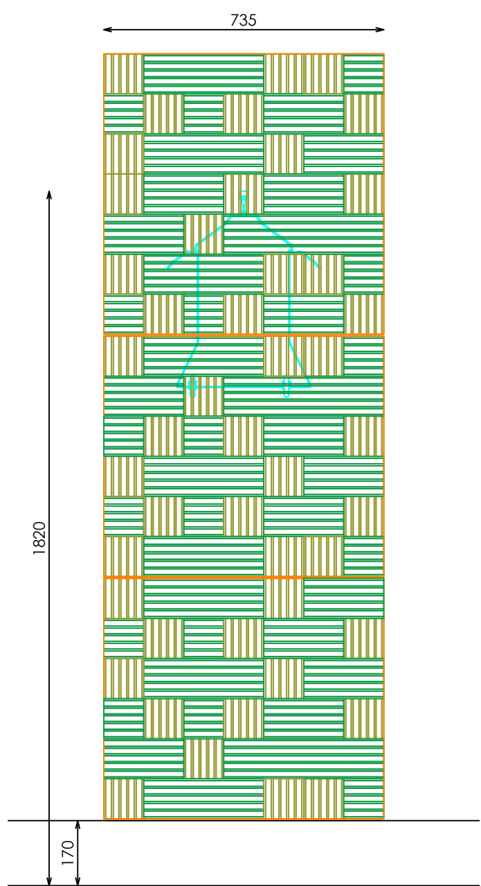
ALZADO FRONTAL
