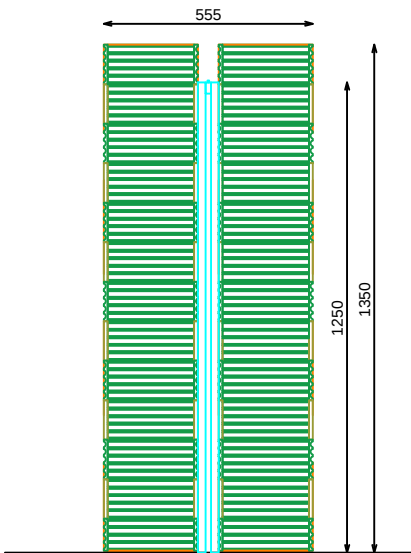
ALZADO LATERAL
