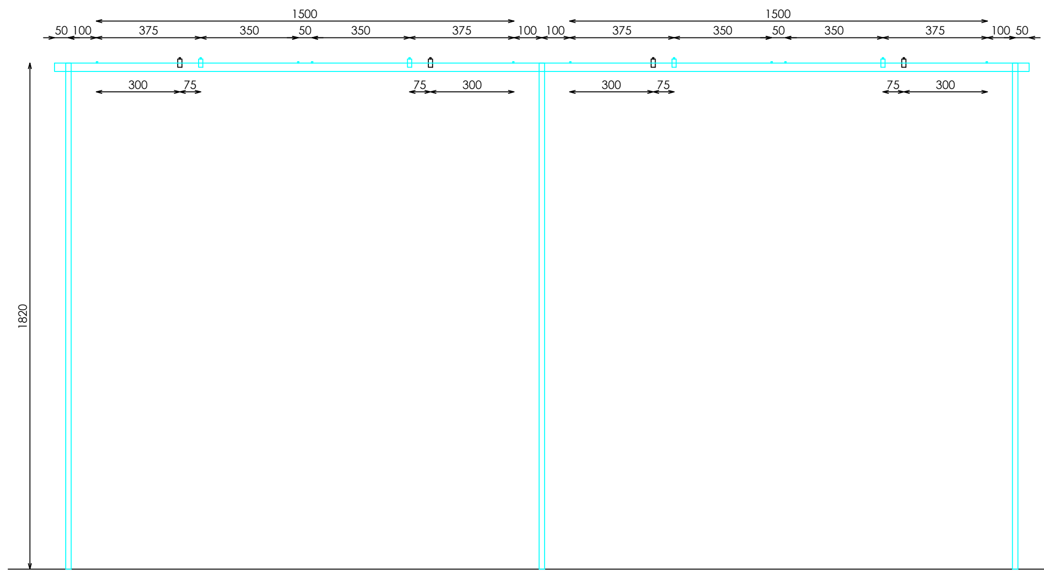
ALZADO
