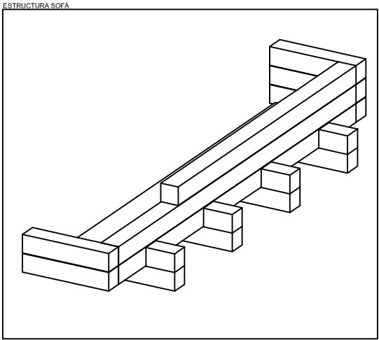
ESTRUCTURA SOFA
