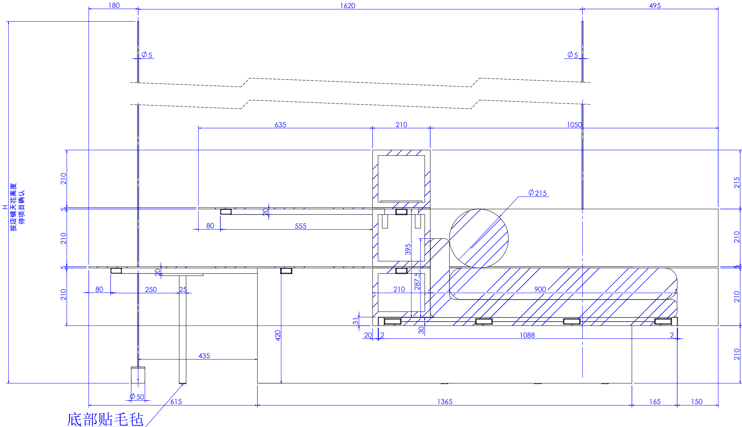
剖面 A-A
