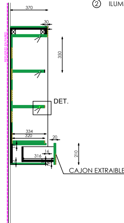
SECCIÓN
