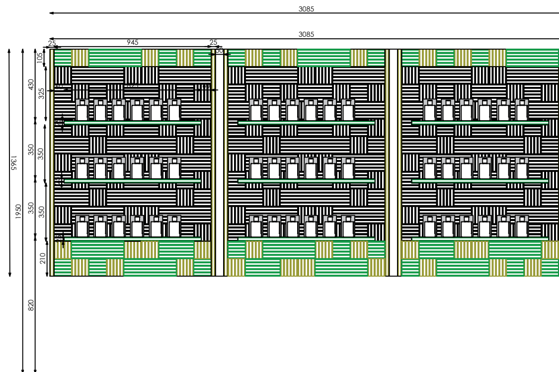
ALZADO FRONTAL
