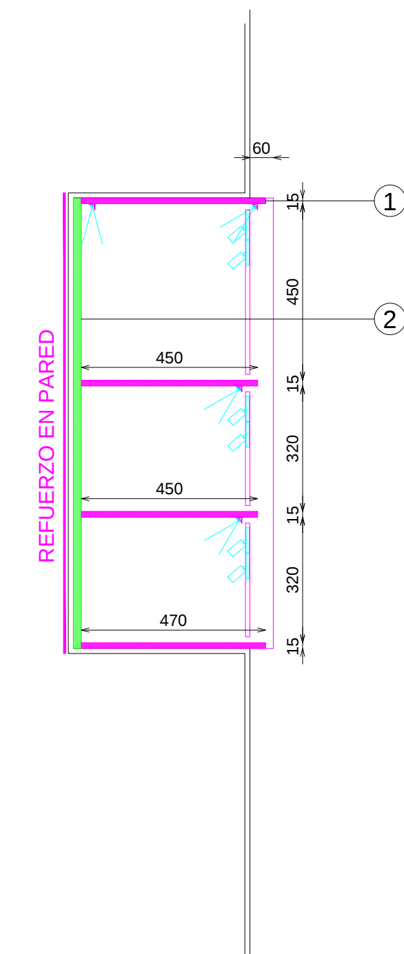
SECCION
